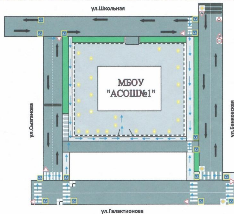
Типовое решение пешеходного перехода расположенного вблизи образовательной организации
